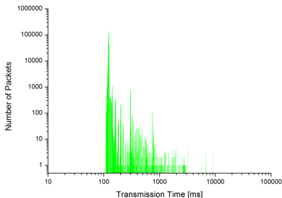
Abbildung 40: GSM Download-Richtung (DIP-DEP) L_{\text{Pkt}}=256 Byte, T_{\text{TI}}=500 ms
