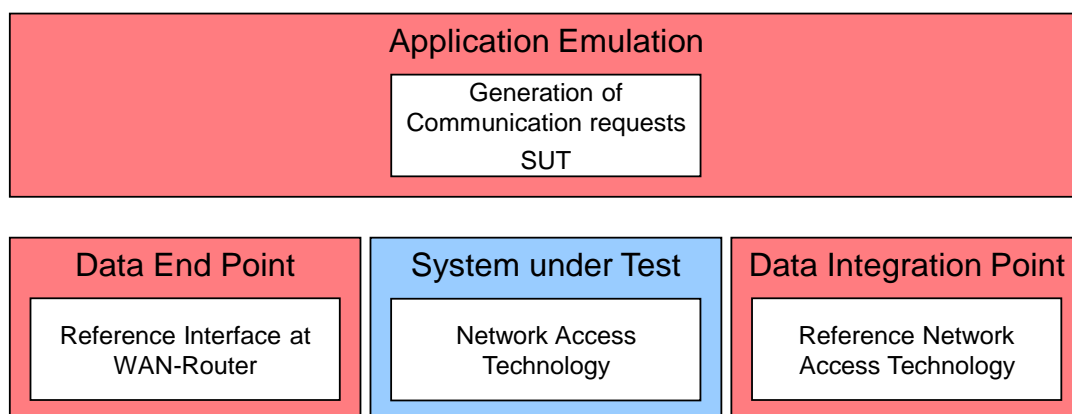
Abbildung 26: Funktionelle Teststruktur
