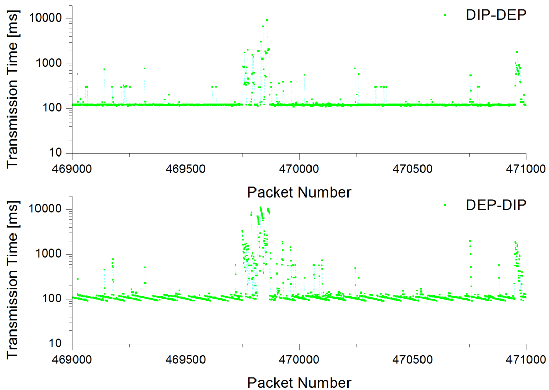
Abbildung 42: Maximale Übertragungszeit (GSM: L_{\text{Pkt}}=256 Byte, T_{\text{TI}}=500 ms)
