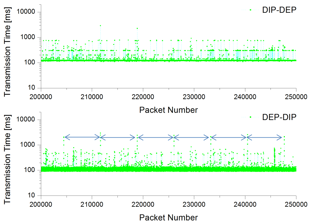
Abbildung 43: Zyklische Ausreißer (GSM: L_{\text{Pkt}}=256 Byte, T_{\text{TI}}=500 ms)
