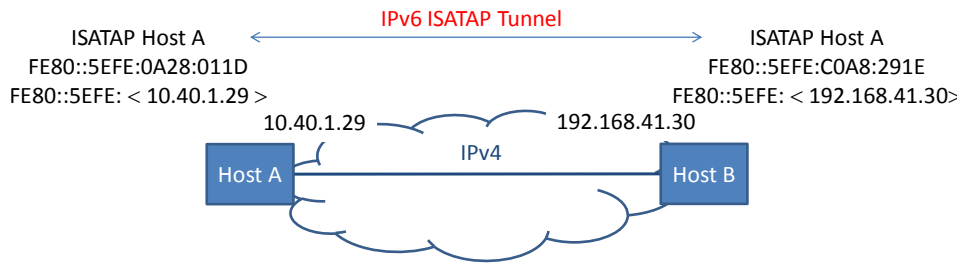
Abbildung 72: ISATAP Konfiguration zwischen zwei IPv6 Host
