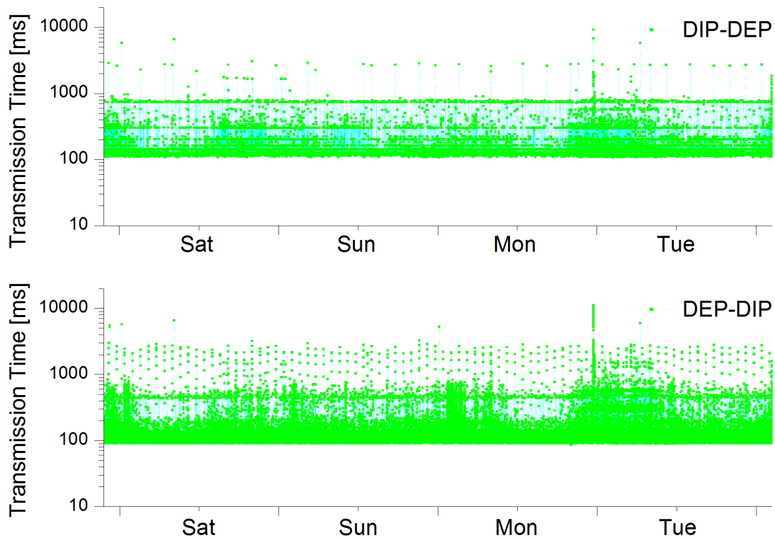
Abbildung 39: GSM Up- und Download-Richtung: L_{\text{Pkt}}=256 Byte, T_{\text{TI}}=500 ms
