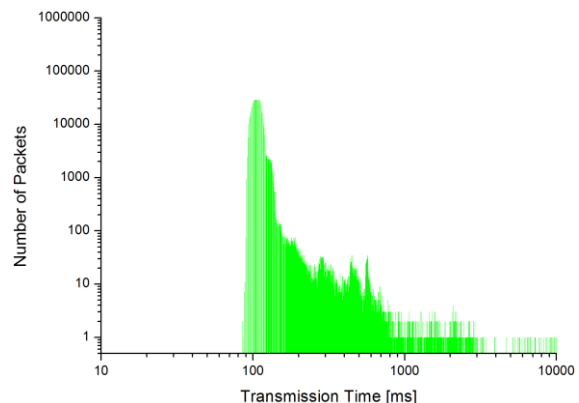
Abbildung 41: GSM Upload-Richtung (DEP-DIP) L_{\text{Pkt}}=256 Byte, T_{\text{TI}}=500 ms
