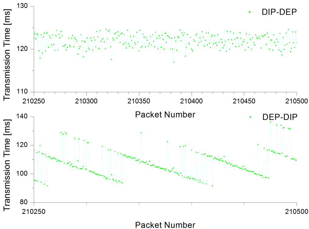
Abbildung 44: Asynchrone zyklische Prozess (GSM: L_{Pkt}=256 Byte, T_{TI}=500 ms)
