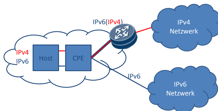
Abbildung 65: Dual-Stack-Lite Architektur
