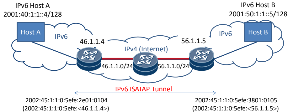
Abbildung 73: ISATAP Tunnel über eine IPv4 Insel
