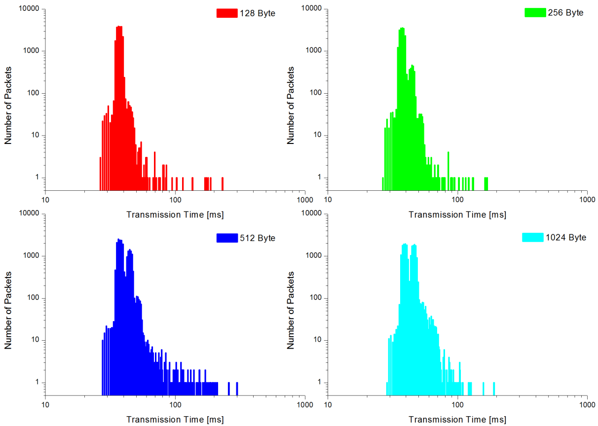
Abbildung 58 LTE: Histogramm der Übertragungszeit T_{TI}=100 ms
