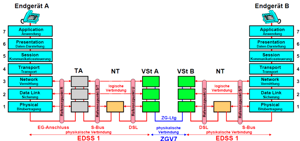
Abbildung 4: ISDN Protokollarchitektur [25]
