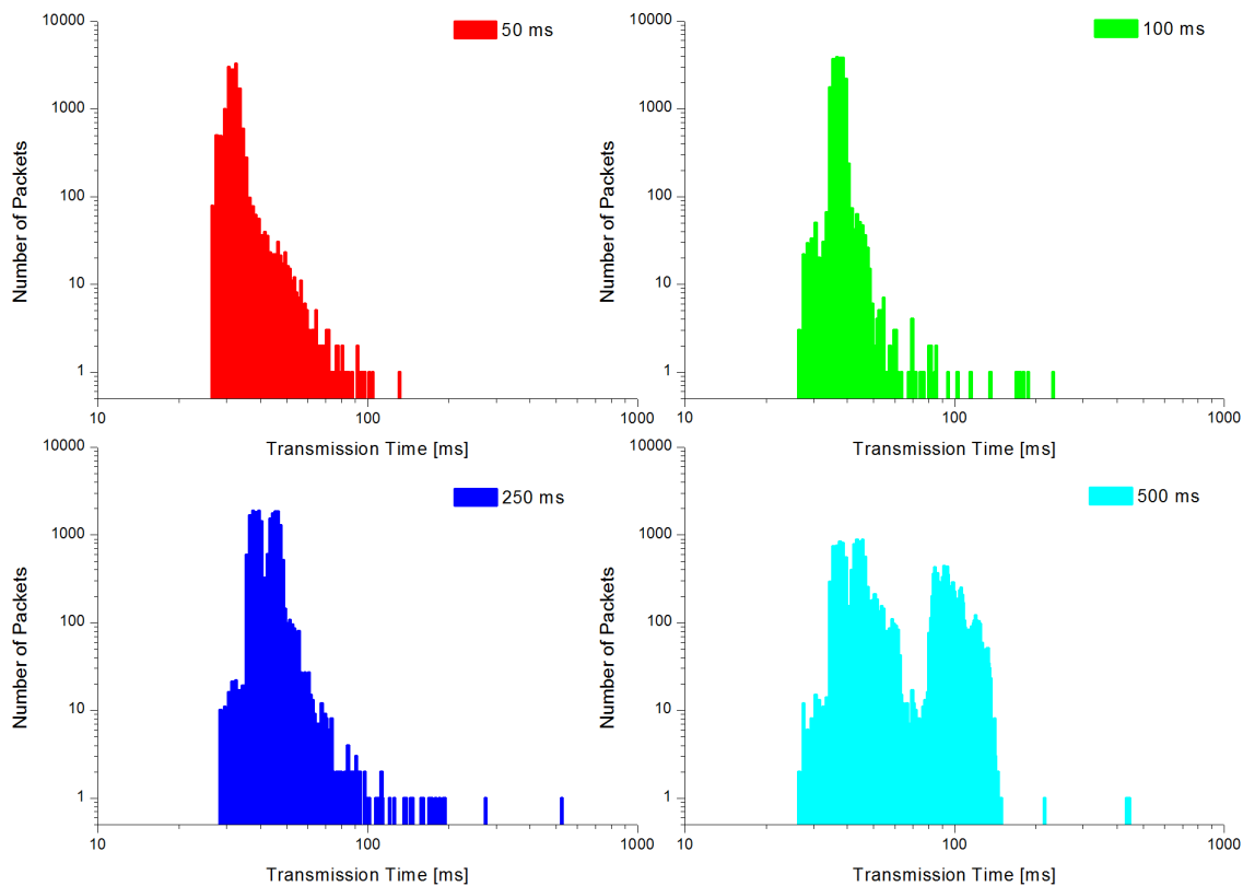
Abbildung 56: LTE: Histogramm der Übertragungszeit für L_{\text{Pkt}} = 128 Byte
