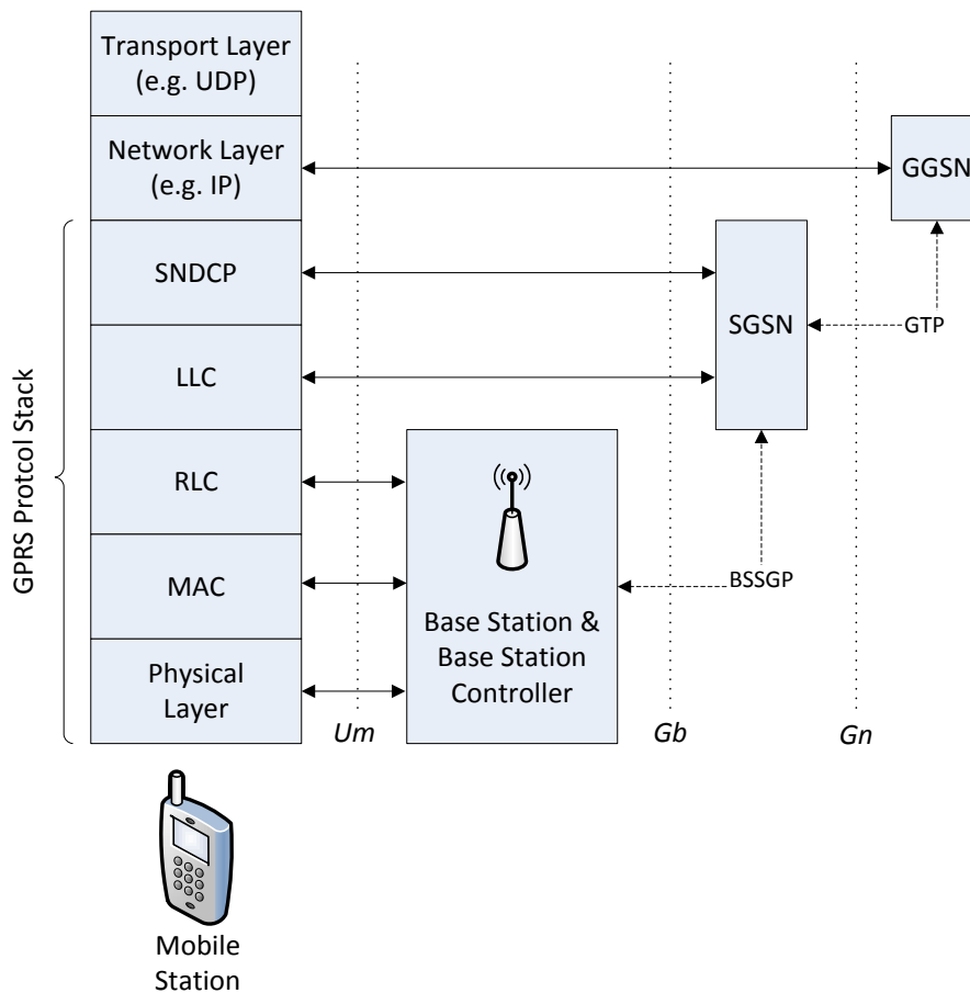
Abbildung 13: GPRS Protokollstack zur Übertragung von Nutzdaten
