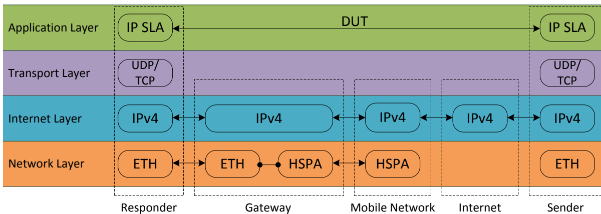
Abbildung 81: Datenpfad der Labortestumgebung aus Protokollperspektive
